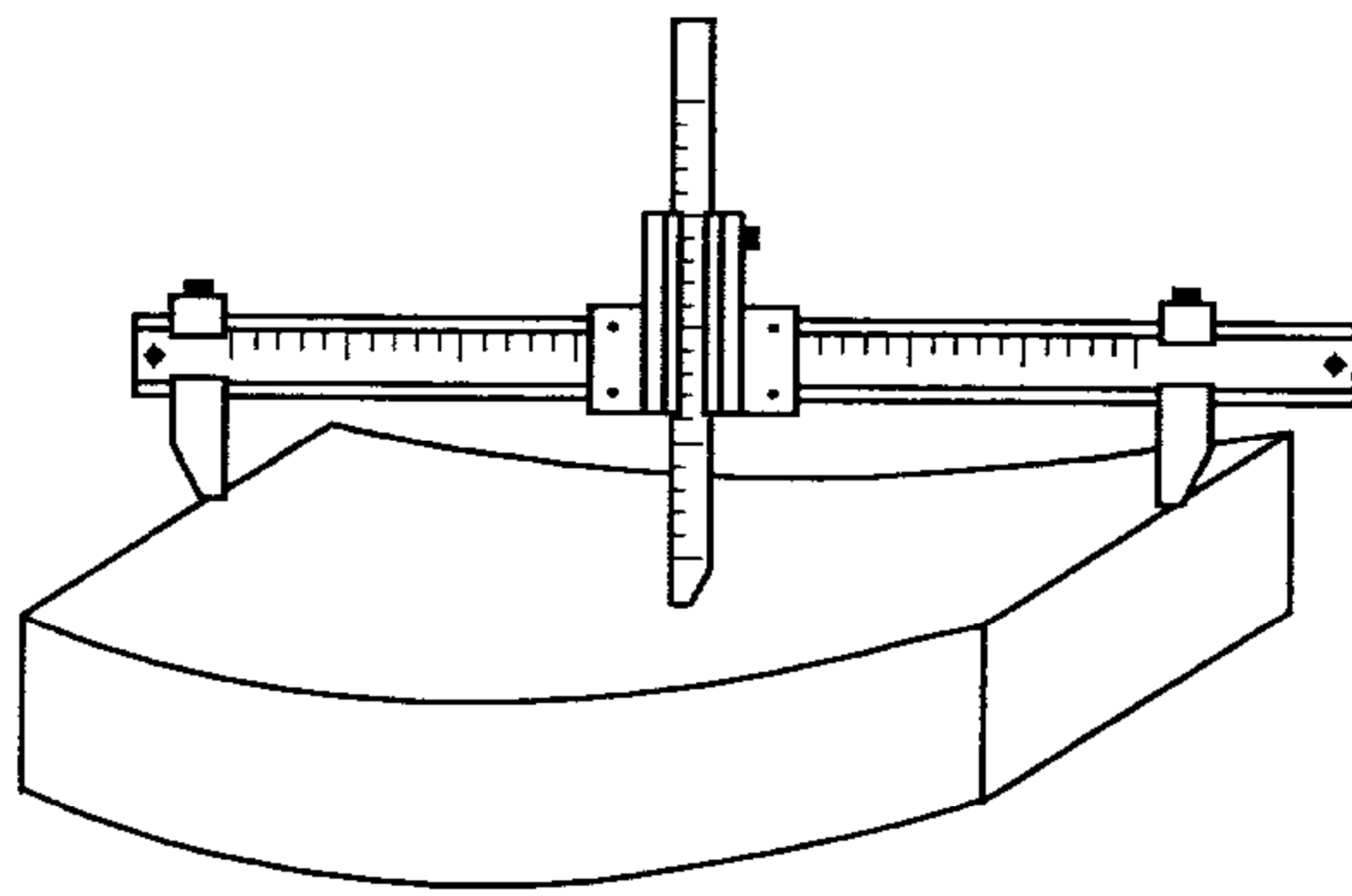
图 7 弯曲量法
