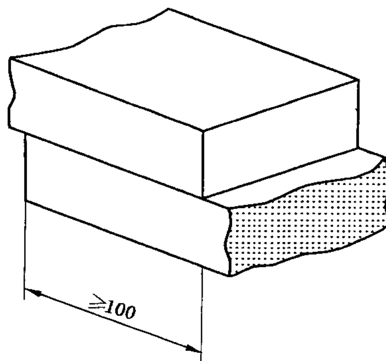
图 12 半砖叠合示意图
