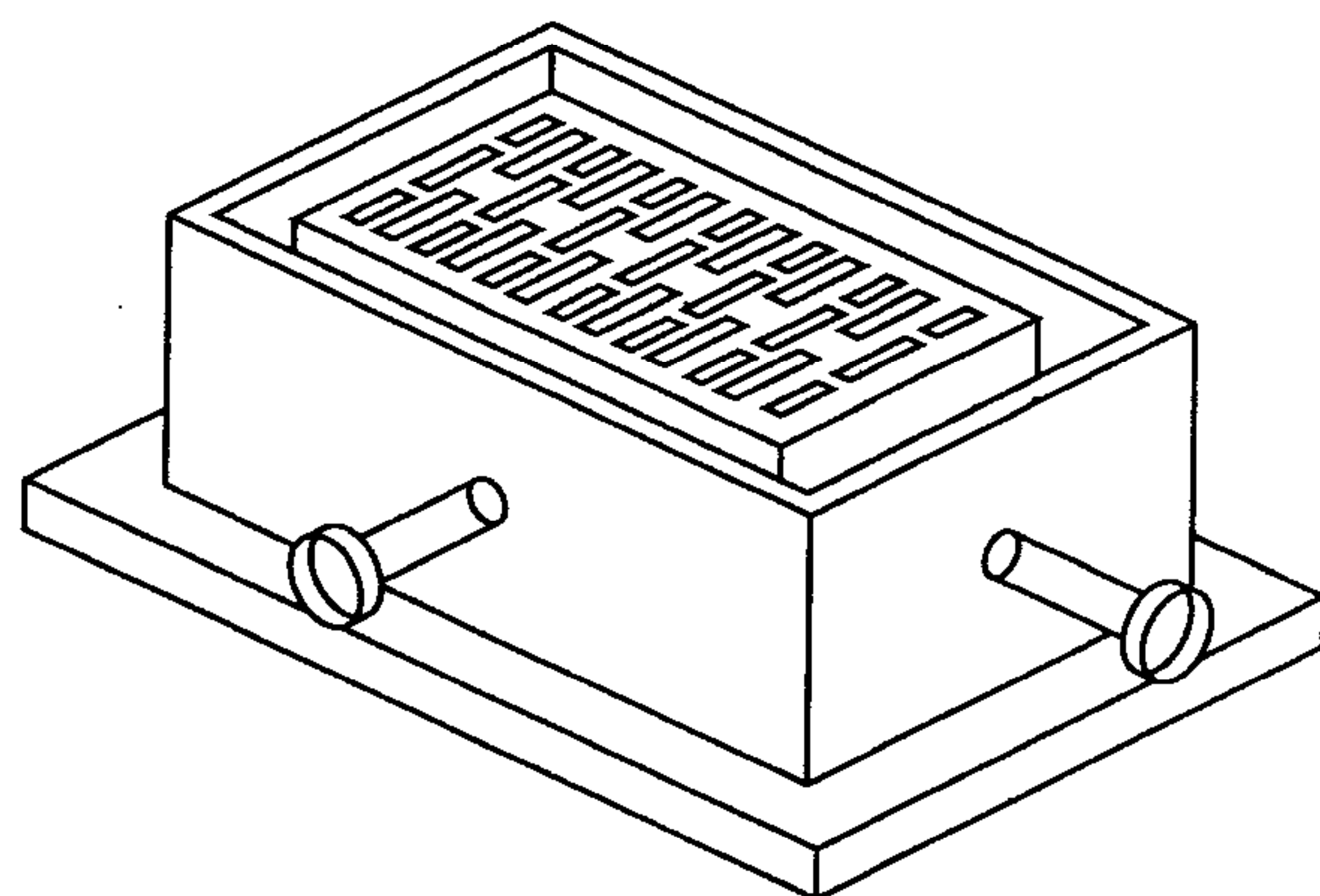
图 11 二次成型制样模具
