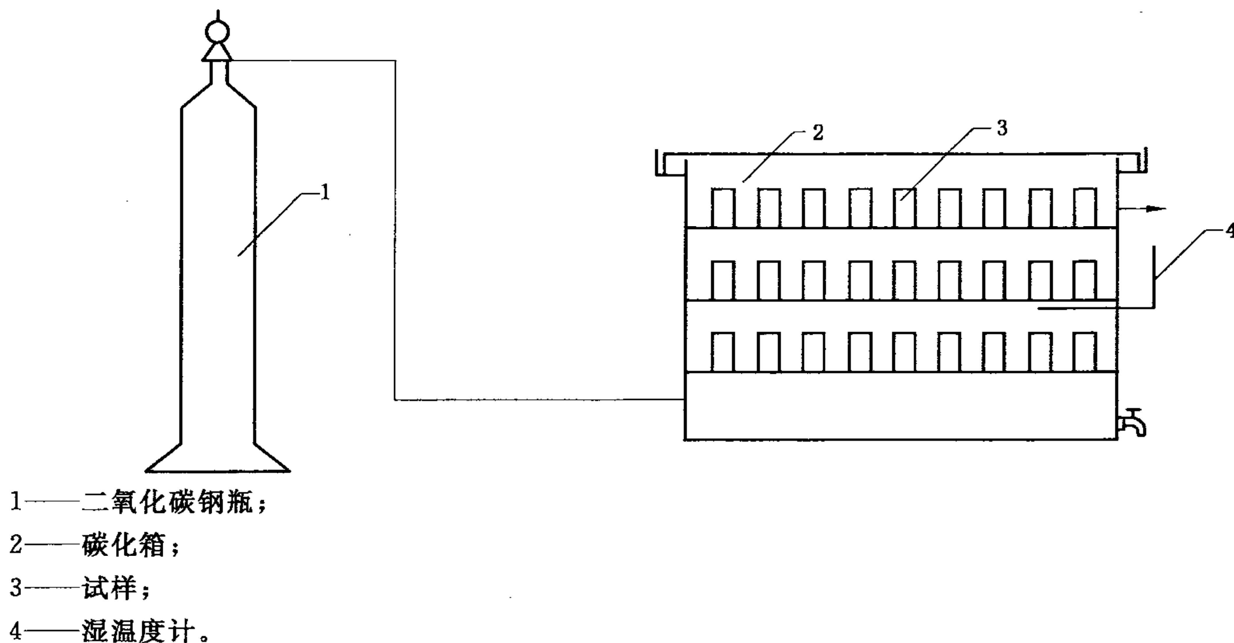
图 16 人工碳化装置示意图
