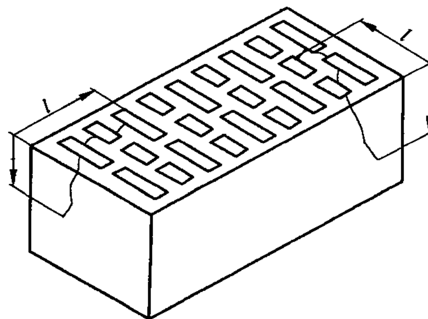
图 6 多孔砖裂纹通过孔洞时长度量法
