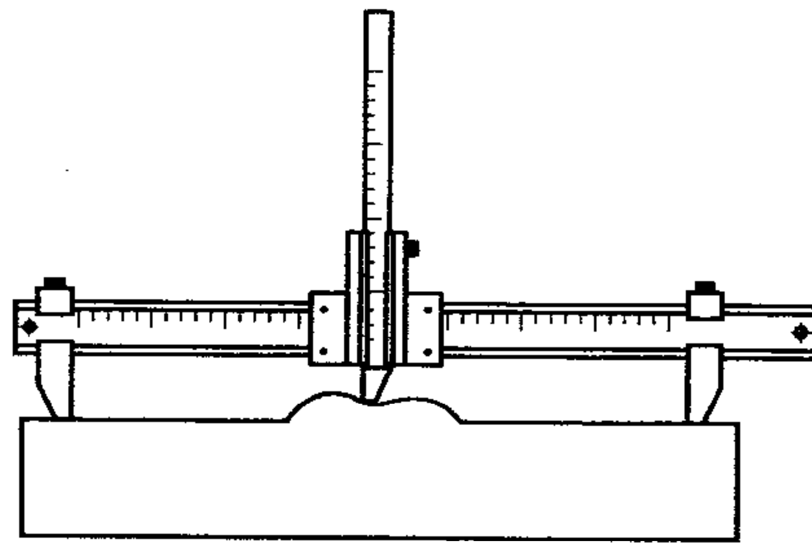
图 8 杂质凸出量法
