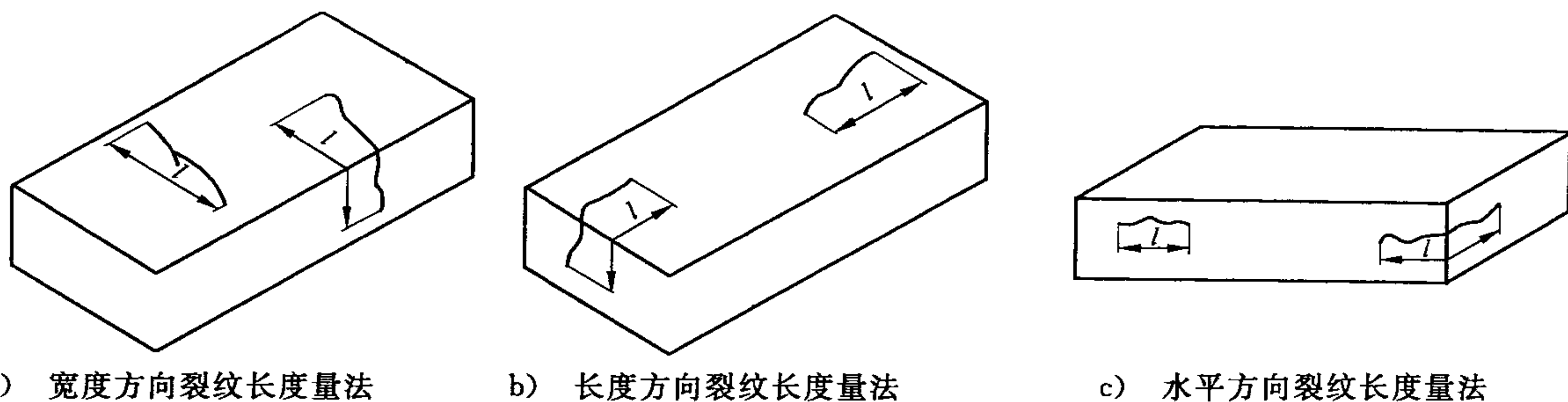
图 5 裂纹长度量法
