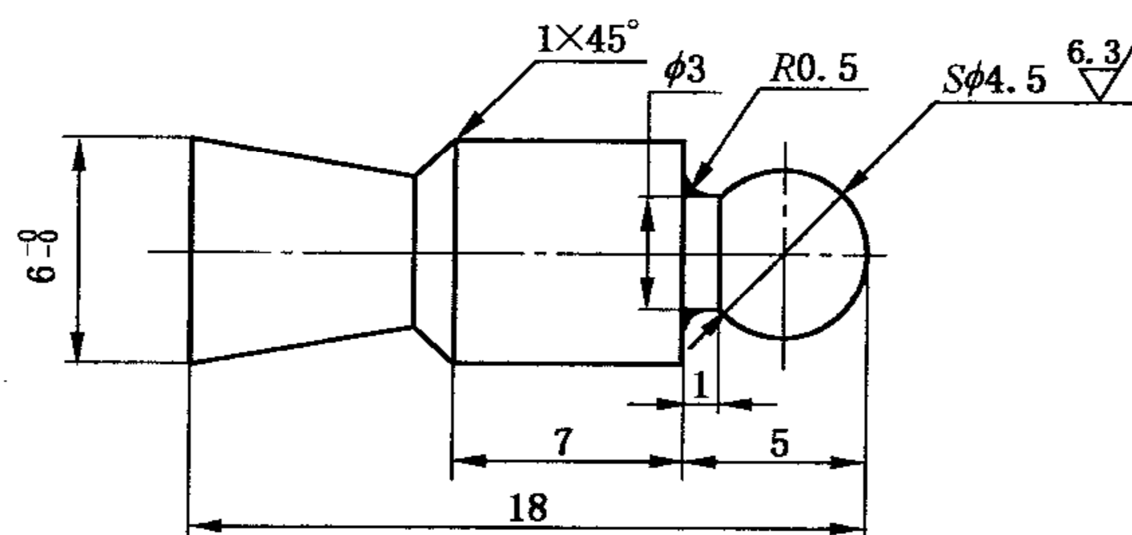
图 15 收缩头
